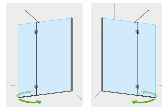
MOD. DESTRO CON TIRANTE DIRITTO APERTURA INTERNO/ESTERNO
