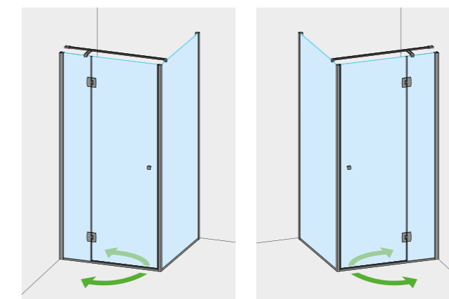
MOD. DESTRO CON MANIGLIA A DESTRA LATI FISSI A DESTRA
