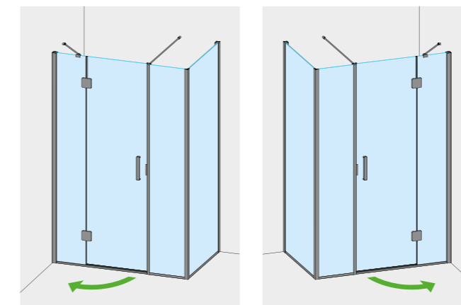
MOD. DESTRO CON MANIGLIA A DESTRA LATO FISSO IN ANGOLO A DESTRA
