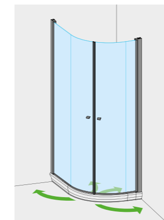
MOD. DESTRO 91X74 CON LATO CORTO A DESTRA
