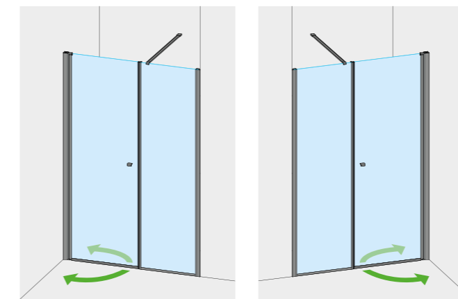
MOD. DESTRO CON MANIGLIA A DESTRA
